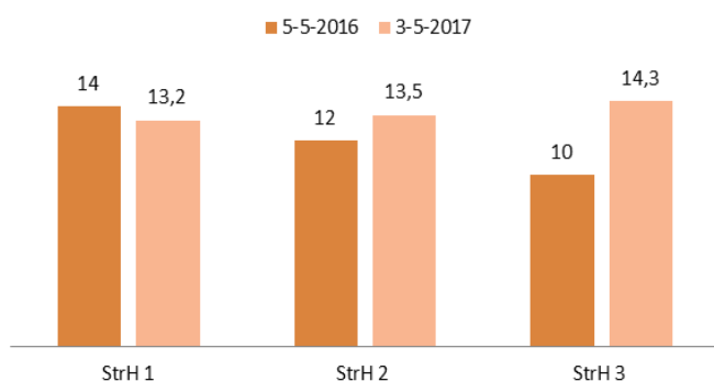
Figuur 6.4: Gemeten watertemperatuur op de drie meetpunten van de Strabrechtse heide op 05-05-2016 en 03-05-2017.
