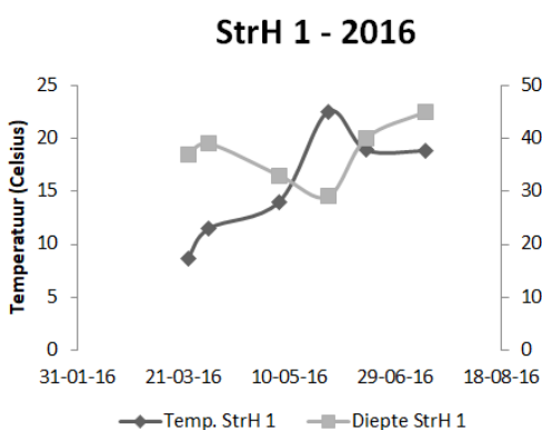
Figuur 6.1: Temperatuur en maximale waterdiepte van meetpunt 1 op de Strabrechtse heide in 2016.
